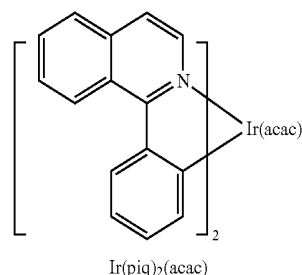
Ir(piq) 2 (acac)
