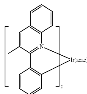
Ir(3-Mepq) 2 (acac)
